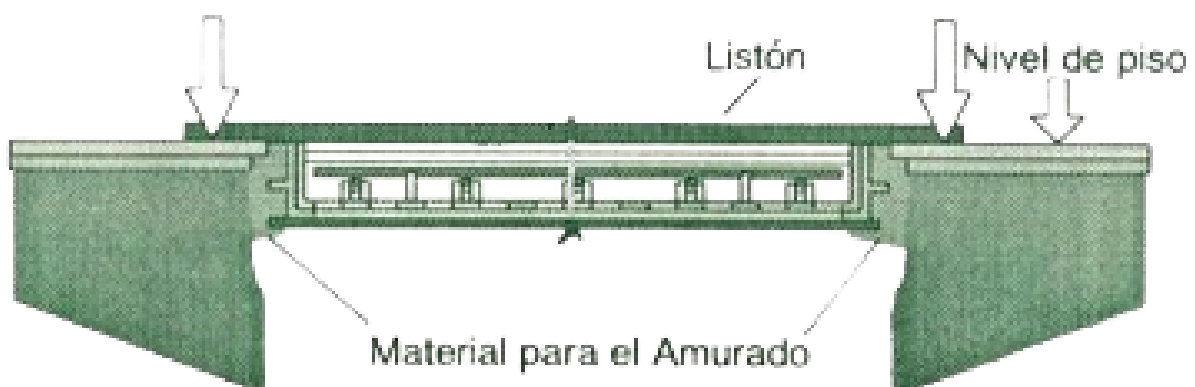
DETALLE DE AMURADO Y TERMINACIÓN
