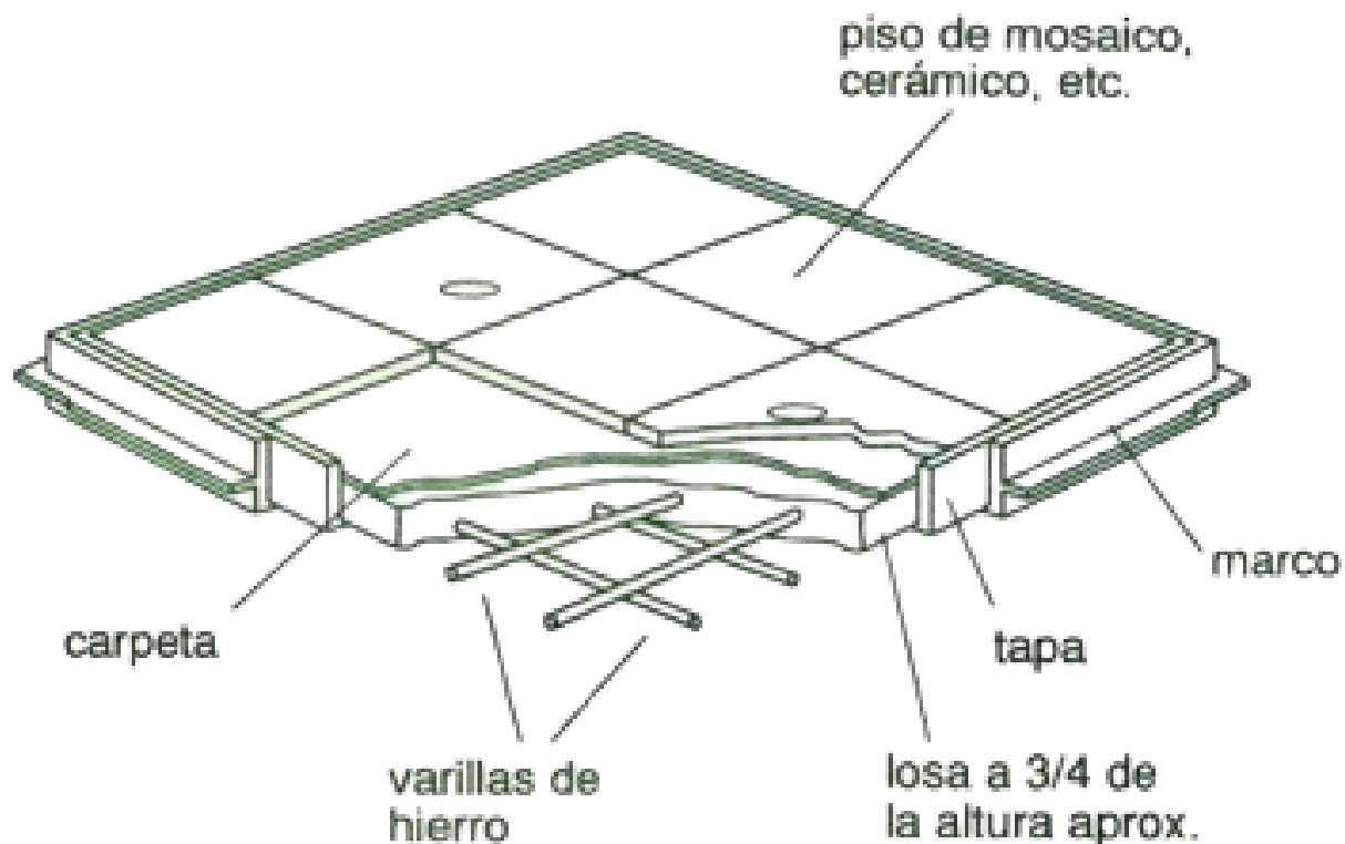
ESQUEMA DETALLADO DE ENCOFRADO
